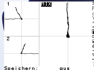
Dual Frequency Mix Mode Gleichzeitige Darstellung beider Prüfkanaäle und des Mixkanals
