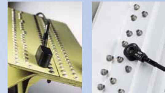
Das ELOTEST M2 V3 ermöglicht alle Arten von Handprüfungen. Von der Hochfrequenz-Oberflächenprüfung an hochlegierten Bauteilen über mittelfrequente Riss- und Korrosionsprüfungen bis zu niederfrequenten Untersuchungen mehrlageriger Strukturen auf Spannungsrisse.
